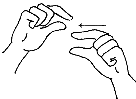
NOUN
